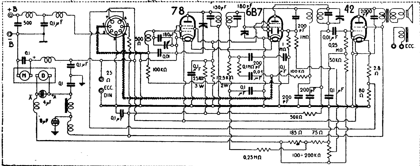
MAGNADYNE - MOD. « AUTORADIO RACI »
